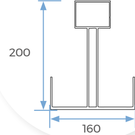
6 TRAVE CENTRALE
