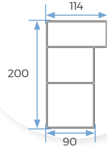
3 TRAVE FRONTALE
