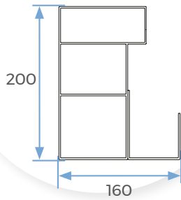
4 TRAVE LATERALE
